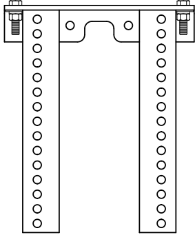
76071 SST estándar Juego para soporte de montaje (para tensor SST XD)
