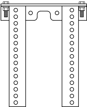
Kit para soporte de montaje estándar (Código del artículo: 76071) • Para la mayoría de instalaciones de limpiador secundario. • 13 x 15-1/2" (325 x 388 mm)
