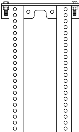
Kit para soporte de montaje prolongado (Código del artículo: 76072) • Para instalaciones que requieren patas extra largas. • 13 x 21-1/2" (325 x 538 mm)
