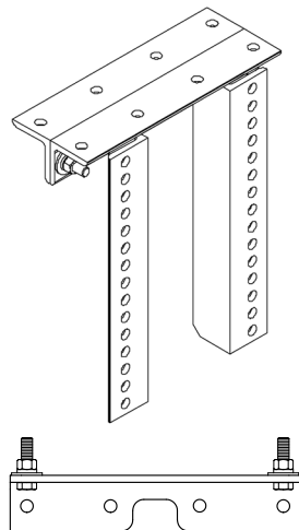
Kit opcional para ángulo superior (Código del artículo: 76073) • Se utiliza con kits para soporte de montaje largo y estándar para opciones de montaje adicional. • 13" (325 mm)
