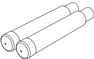
Kit extensor de eje (incluye 2 extensores de eje) (Código del artículo: 76024) • Para tamaños limpiadores de 72" (1800 mm) y mayores. • Proporciona 30" (750 mm) de longitud extendida de eje.
