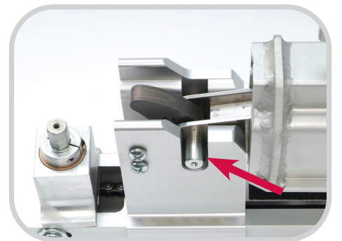
Den Klemmbalken in seine Position fallen lassen
