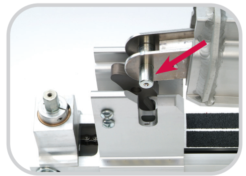
Den Klemmbalken über den Aufnahmen ausrichten
