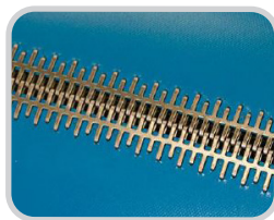
Präzises Stanzen sorgt für eine konstante Teilung von 4,00 mm über die gesamte Länge der Verbindung und für eine einfachere Montage
