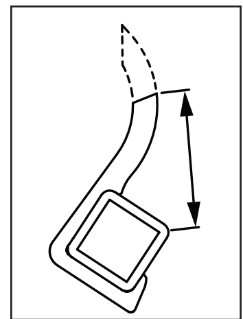
Blattverschleißmessung mit Maßband Blattspitze zur Ecke der Steckachse
