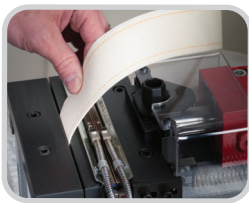
Die integrierte, nicht beheizte Nachpresszone stellt die korrekte Verbindung des Patchmaterials mit dem Wäschereiband sicher
