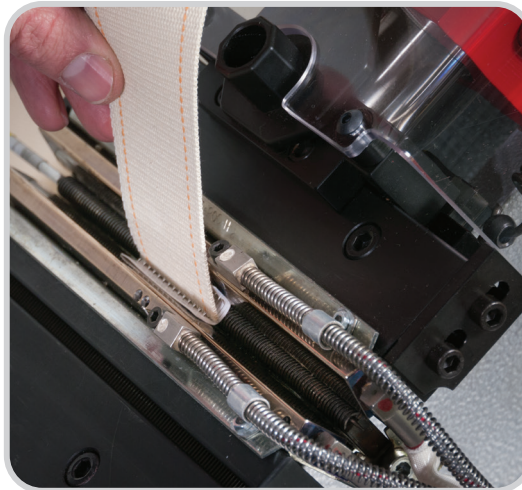
Die integrierte, nicht beheizte Nachpresszone stellt die korrekte Verbindung des Patchmaterials mit dem Wäschereiband sicher
