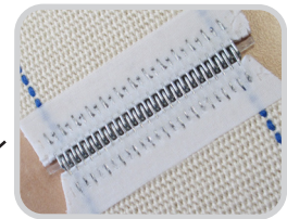
Die Verbinderspitzen sind beim Einpressen durch das Patchmaterial abgedeckt
