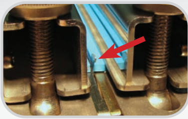
内蔵型カッター: 切断中、刃からオペレーターを保護します。
