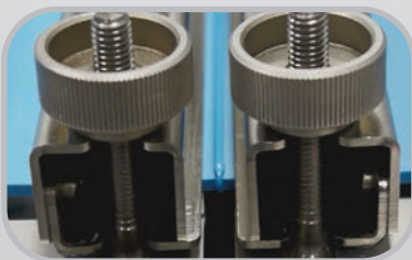
冷却ゾーン: ベルトの端が突き合せ溶接される間にヒーターを収容し、本体の中で冷却します。
