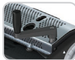
La zona de calentamiento protegida y control de temperatura garantizan la consistencia de los parámetros de empalme independientemente de las temperaturas ambientales
