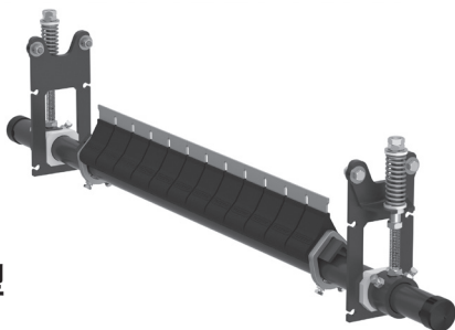
Y-Type™ 标准型 (带碳化钨刮刀)
