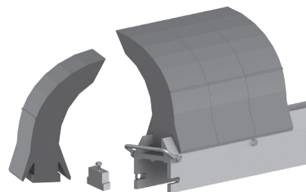
刮刀架组件
