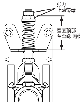
上拉张紧装置配置 (HD)
