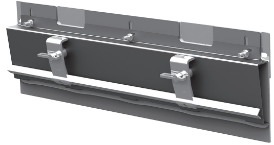
带 6 mm (1/4") AR400 的切线型护衬组件
