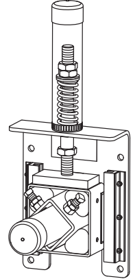
二级清扫器张紧装置上的弹簧盖
