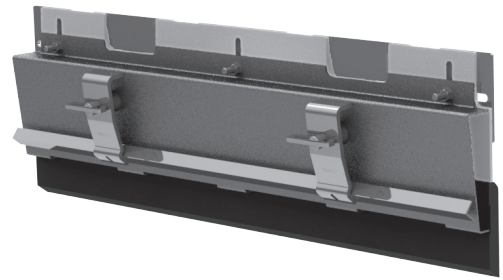
带 25 mm (1") 船形护衬的切线型护衬组件
