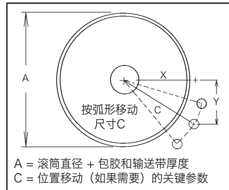
固定杆位置规格
