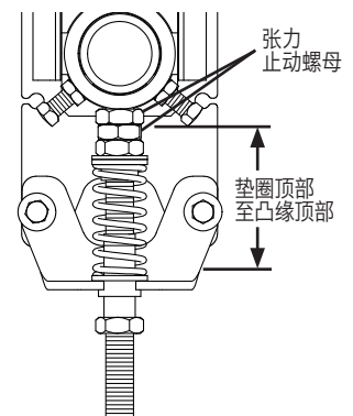
上推张紧装置配置 (HD)
