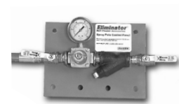
喷水固定杆控制板
