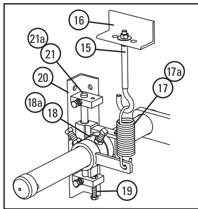
用于将 UST 弹簧张紧装置更换为钩头螺栓张紧装置
