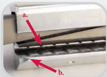
Der untere Keil mit Rippen und das Gehäuse mit Nute bieten zusätzliche Haltekraft (a.).
