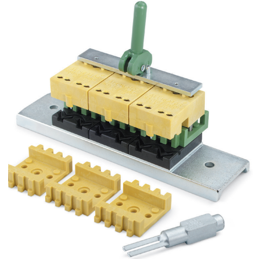
Montagewerkzeug RSC187
