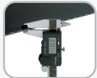
Banddicke messen
