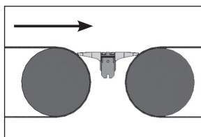
Für Bandanwendungen horizontal nach horizontal. Den Abstand zwischen den Trommeln an einem Punkt messen, der nicht mehr als 25 % des Trommeldurchmessers (einschließlich Dicke des Bands) tiefer als die Oberseite beider Trommeln ist.
