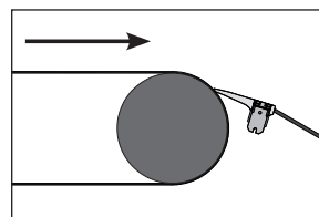
Für Übergänge von Band zu Übergabetrichter oder Rutsche. Auf der Trommelseite nicht höher als 13 mm unter der Oberseite und das Brückensegment ca. 4 bis 13 mm über dem Übergabetrichter oder der Rückseite der Rutsche.
