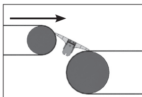
Für „Wasserfall“-Anwendungen. Den Abstand zwischen ca. 45° vom höchsten Punkt der oberen Trommel zum höchsten Punkt der unteren Trommel messen.
