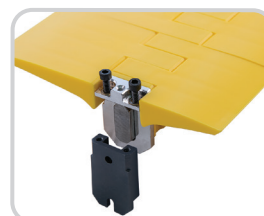
Einfach zu montieren und zu entfernen durch den zweiteiligen Montagehalter.
