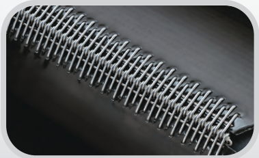
Drahtaken-Verbindungssystem Clipper®
