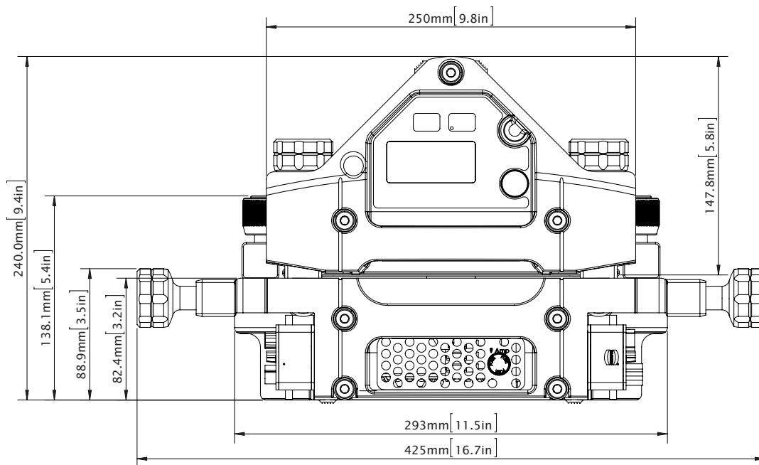
Vista delantera y medidas de las prensas Aero®, tamaños 625-1225.
