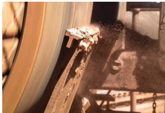
Se muestra: Prelimpiador hoja V-TIP tipo H
